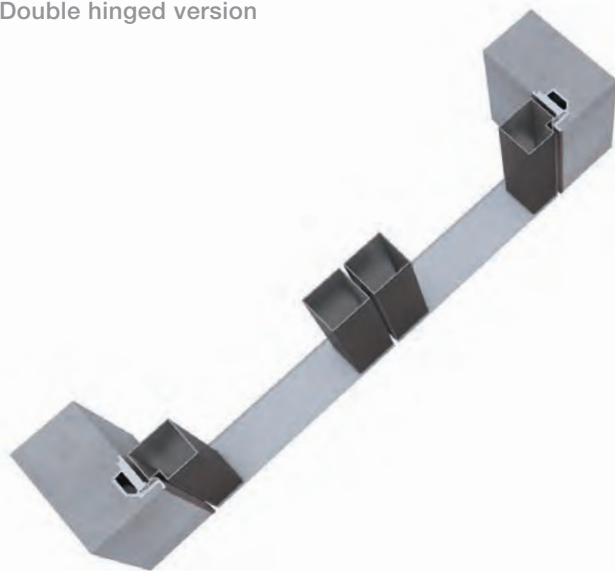
FILOMURO CRYSTAL Versione doppio battente Double hinged version
