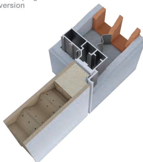
FILOMURO PLUS PER MURATURA / MASONRY Versione a spingere Push version
