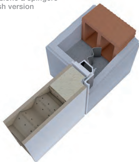
FILOMURO MINIMA PER MURATURA / MASONRY Versione a spingere Push version
