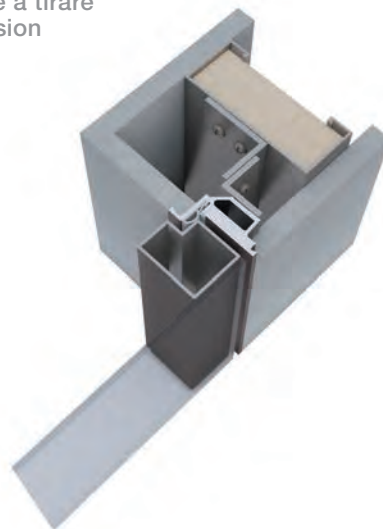
Versione a tirare Pull version
